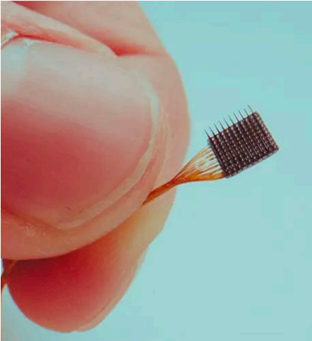
Utah Array
